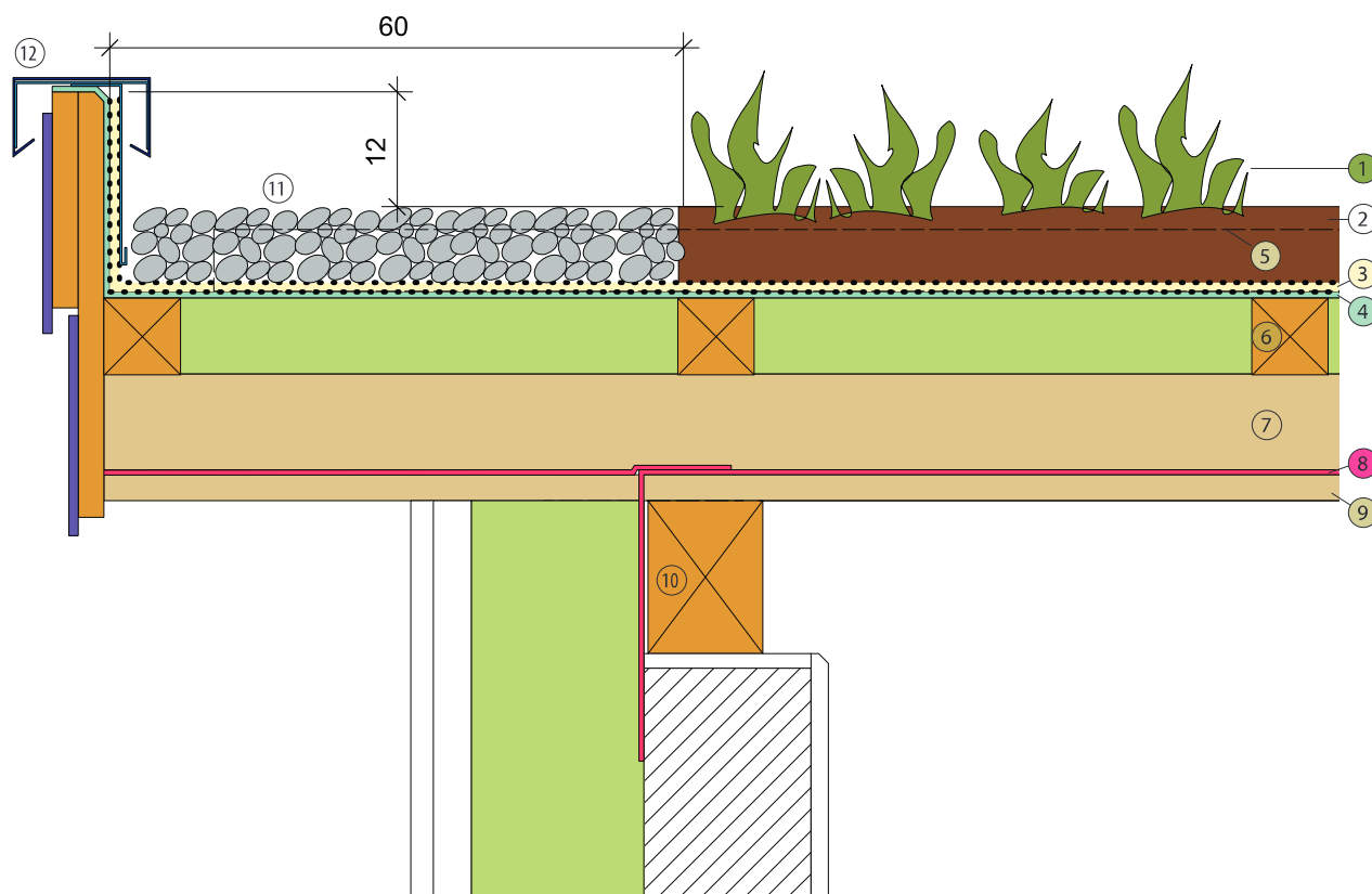
Abb.: Dachaufbau Dachbegrünung, Ortgang
